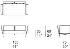
Divano due posti / 2-seater sofa B198CA
